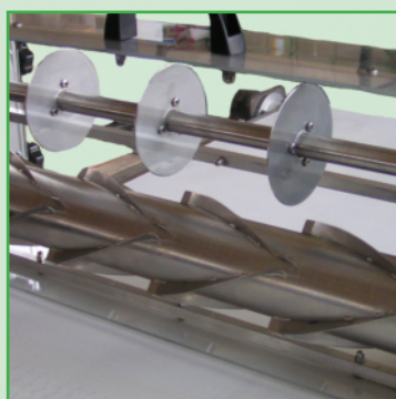
Stazione di taglio Cutting set Ensemble de coupe Juego de corte
